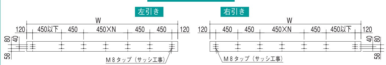
寸法図
