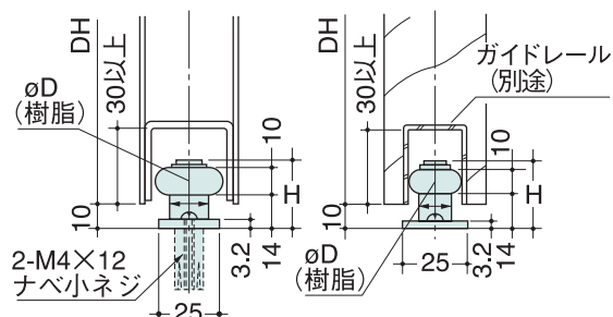
サッシ扉
