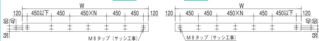
寸法図
