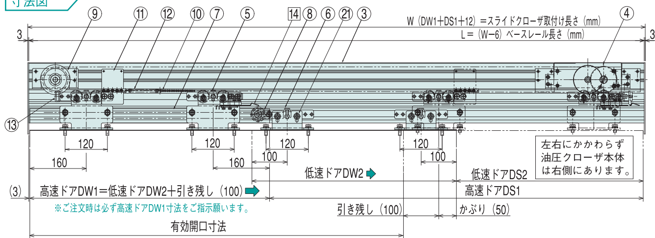
寸法図
